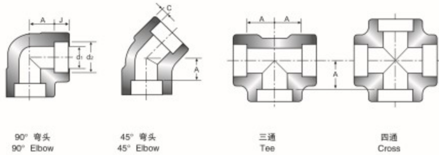
承插焊管件 (一) Socket Welding Fittings GB/T 14383、SH3410、ASME B16.11
